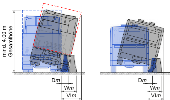
Darstellung 3: Grundlagen zum Wirkungsbereich und zur Fahrzeug-Eindringtiefe
