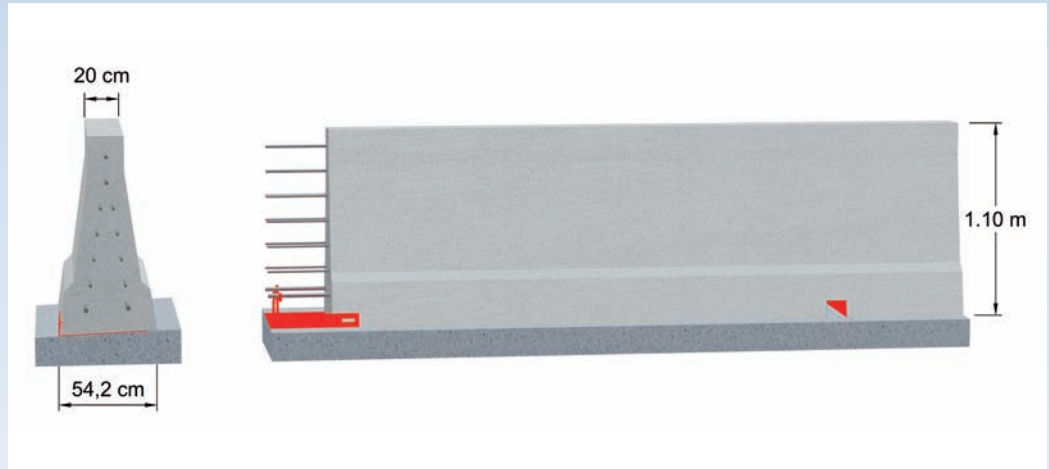
Bild 2: Die Ortbetonschutzwand LT 104, hier in der Variante für Bauwerke, bietet mit der Aufhaltestufe H4b höchste Sicherheit. Ein umfangreiches Programm an Modulen sowie an Übergangskonstruktionen und -elementen erlaubt den Anschluss an andere Betonschutzwände sowie an Stahlschutzplanken
